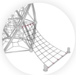
1 Наклонная сетка
